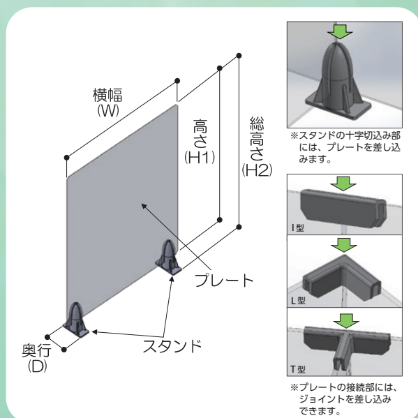
ジョイント部品 (ABS)
