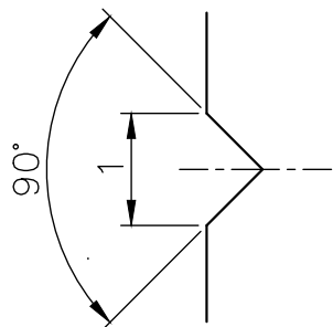
φa及びφb寸法の溝形状
