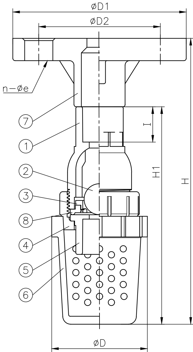
フランジ式
